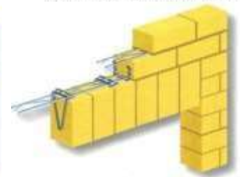
ВЕРТИКАЛЬНАЯ КЛАДКА
